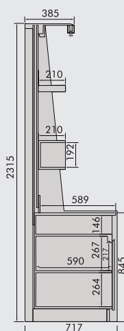
Retro Modular Tetris C/Módulo Portas
