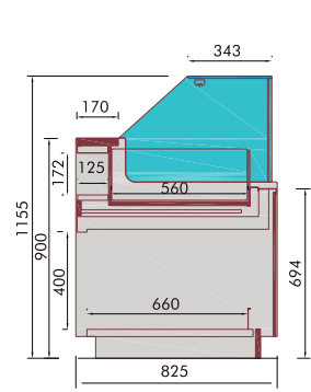
Bellini Pão VVRB
