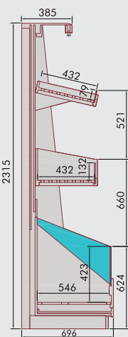
Retro Modular Tetris C/Módulo Tulha
