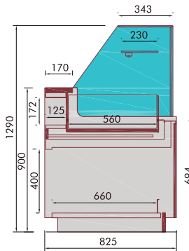
Bellini Pão VVR
