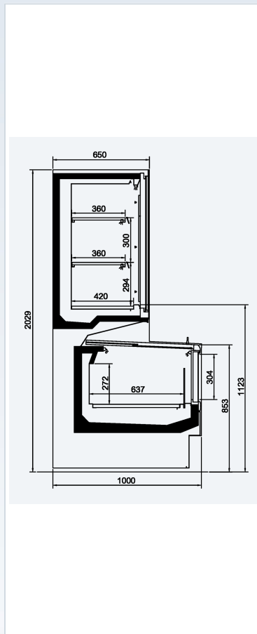
COUPE COTÉE (MM)
