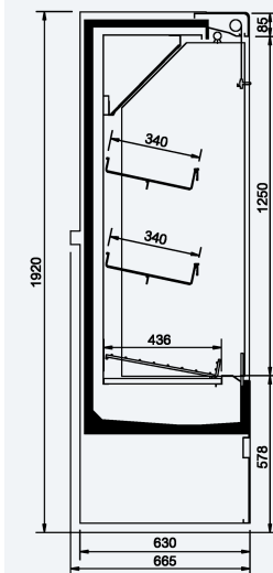
COUPE COTÉE (MM)
