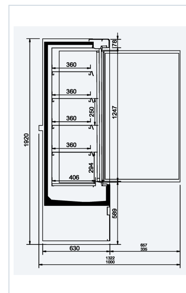
COUPE COTÉE (MM)
