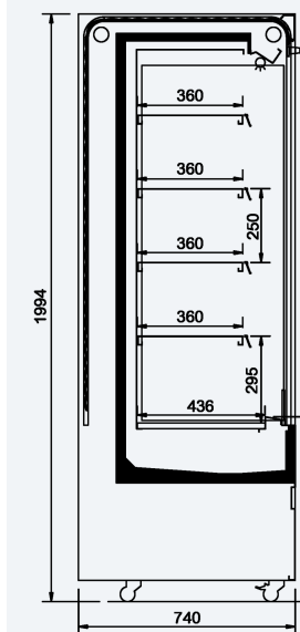
COUPE COTÉE (MM)
