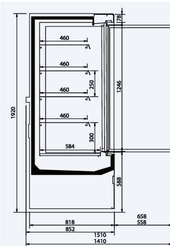
COUPE COTÉE (MM)
