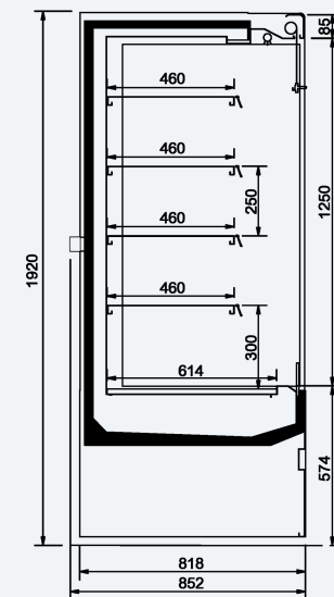
COUPE COTÉE (MM)
