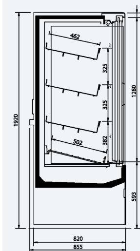
COUPE COTÉE (MM)
