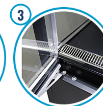
REPRISE D'AIR 5 niveaux réglables sans grille et goulotte inox en façade
