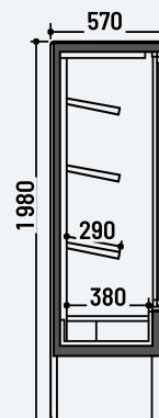
ÉTAGÈRES INCLINABLES
