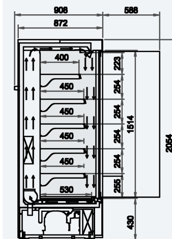
COUPE COTÉE (MM)
